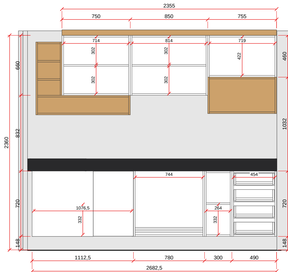
VISTA A - ESC. 1:25
