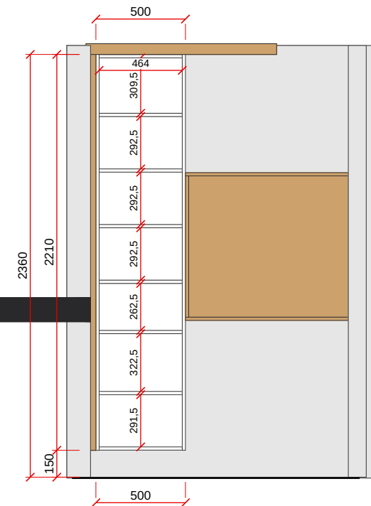
VISTA D - ESC. 1:30
